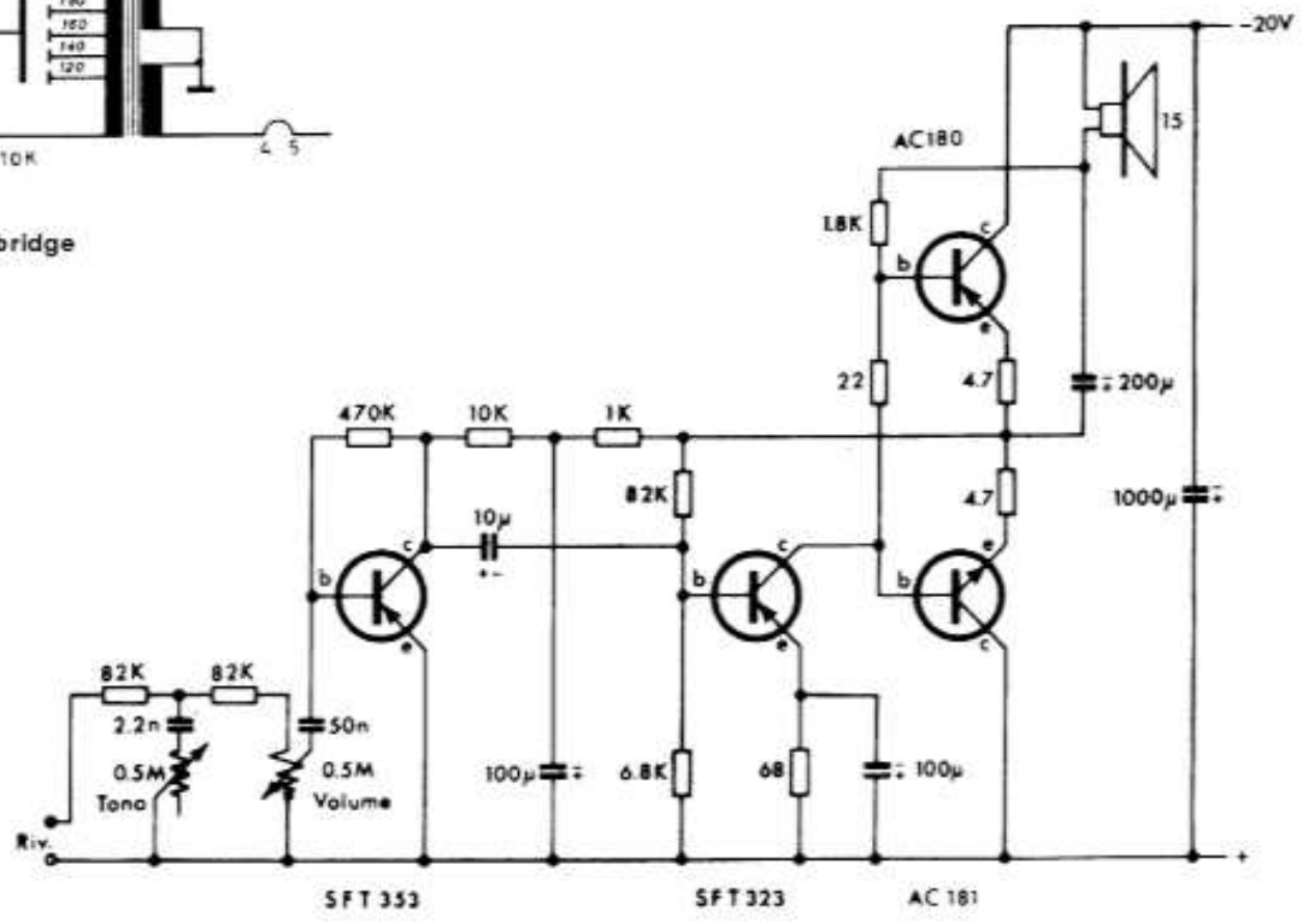
SCHEMA ELETTRICO DELLE FONOVALGIE G.B.C. FV/4 CAMBRIDGE X e FV/9 MIKE
